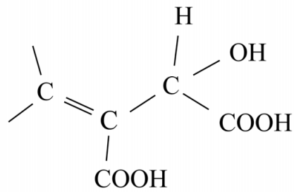
trans -hydroxyaconietzuur
